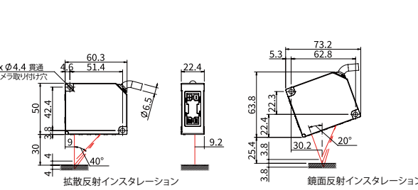
SD33-30-485-□-△
