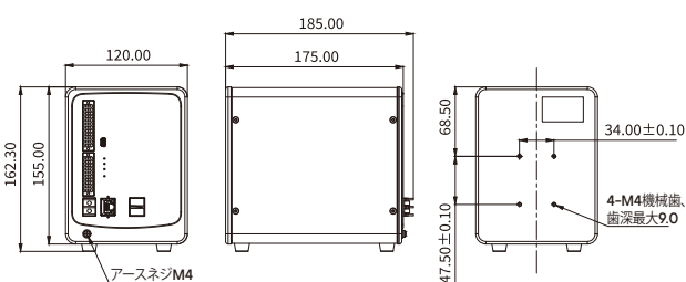
SCI501A/SCI501B 一対一
