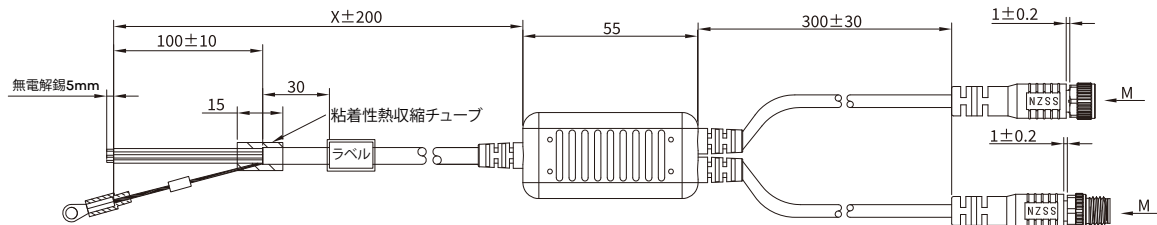
Y型ケーブル SCB-EY-HB2-Xm
