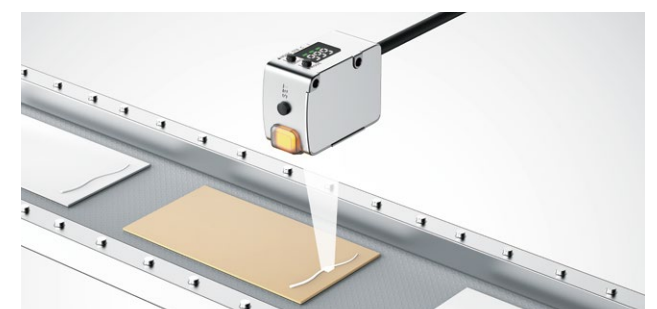
接着剤検出
