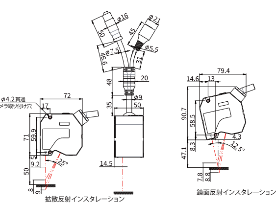
SGI050 SGI055
