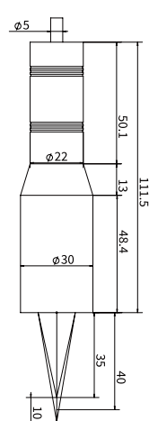
SCI10015
