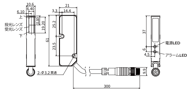
受信センサーヘッド SE1-010K4-R
