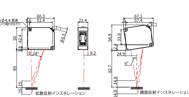
SD33-85-485-□-△
