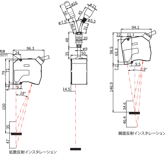
SGI150 SGI155
