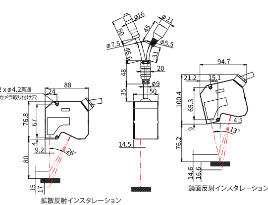
SGI080 SGI085
