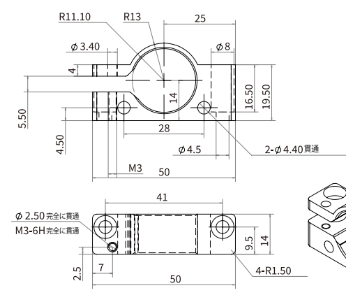
SCI-01
