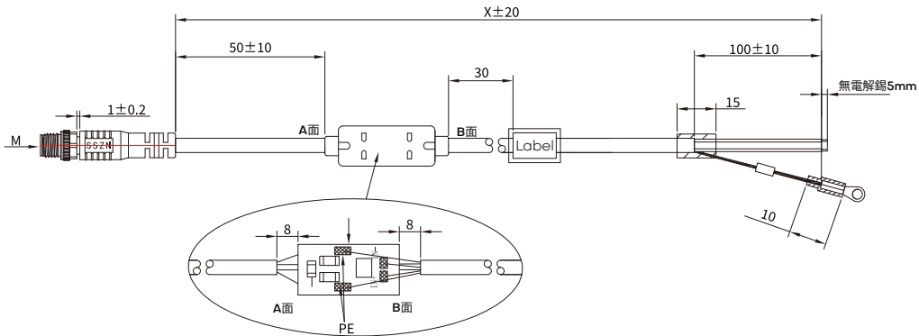
電源ケーブル SCB-EPWR-HB4-Xm
